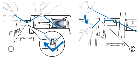
① Przewodnik nici ② Pokrywa przewodnika nici
