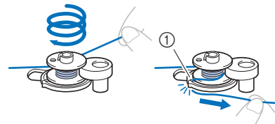
① Szczelina prowadząca w gnieździe nawijacza szpulki dolnej (z wbudowanym przecinakiem)
