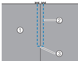
① Wierzchnia strona tkaniny ② Ścieg ③ Koniec otworu zamka
