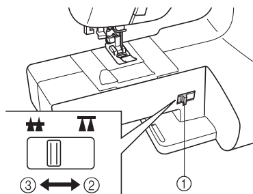
① Przełącznik pozycji transporterów ② Pozycja dolna ③ Pozycja górna
