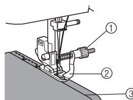
① Śruba ② Prowadnik ③ Zagięty brzeg
